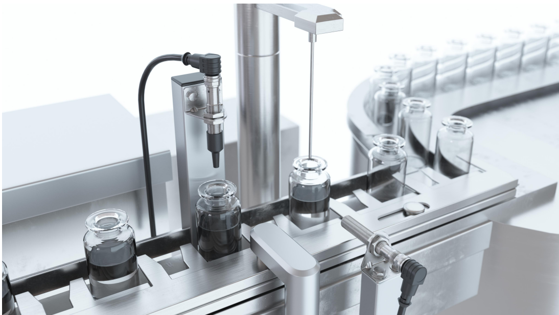
Ultraschallsensoren der Reihe UT12 in einer automatisierten Dosieranlage: Das Gerät hinter der Dosiereinheit kontrolliert von oben die Füllstände durch die kleinen Flaschenöffnungen. Ein weiterer Sensor mit Schaltausgang dient zur Anwesenheitskontrolle. (Alle Bilder: ipf electronic)
