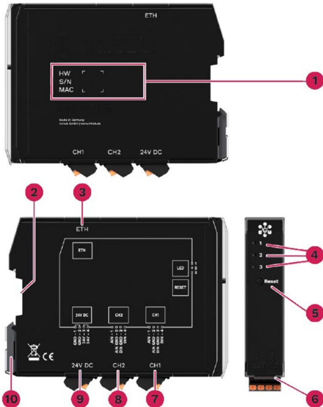
Abb. 2: Seitenansichten und Vorderansicht des AB000010 inkl. Schnittstellen
