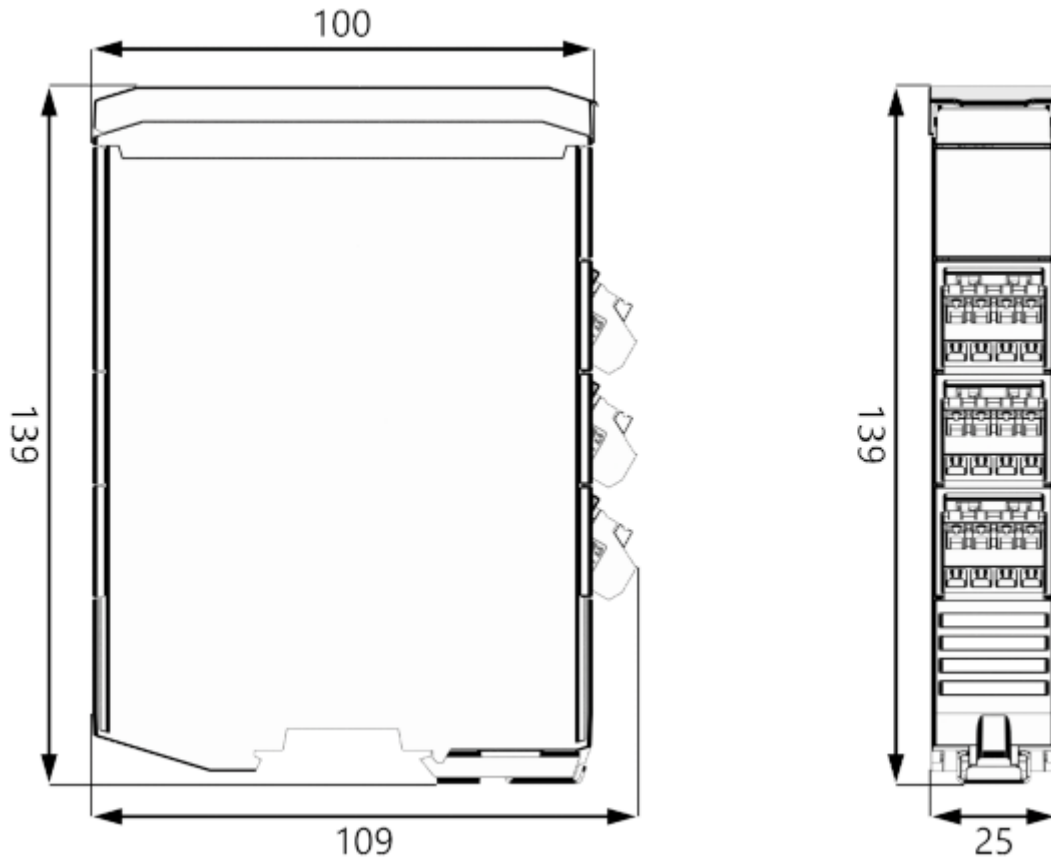
Abb. 8: Schematische Zeichnung des AB000010 (Maße in mm)
