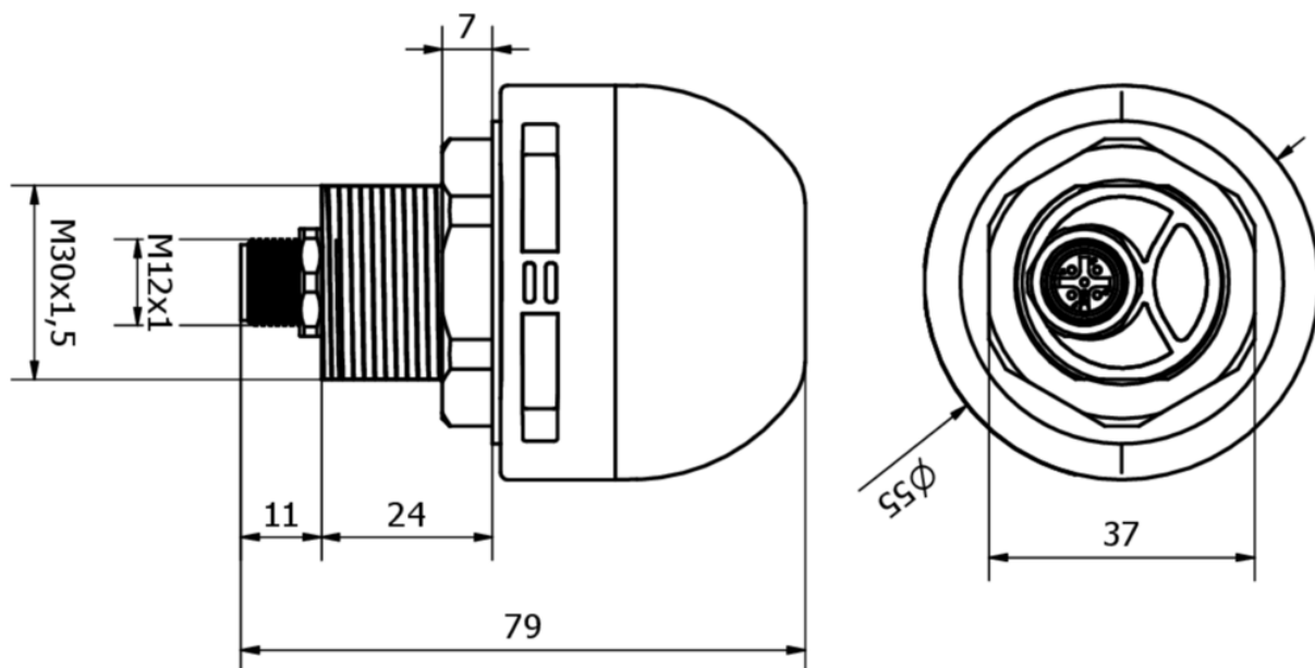
Maßskizze EZ550320
