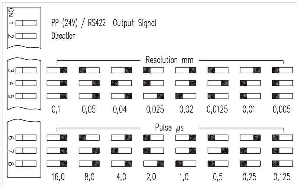
Abb. 2: DIP-Schalter-Einstellungen
