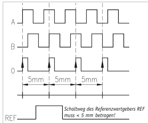
Abb. 4: Prinzip der Referenzierung
