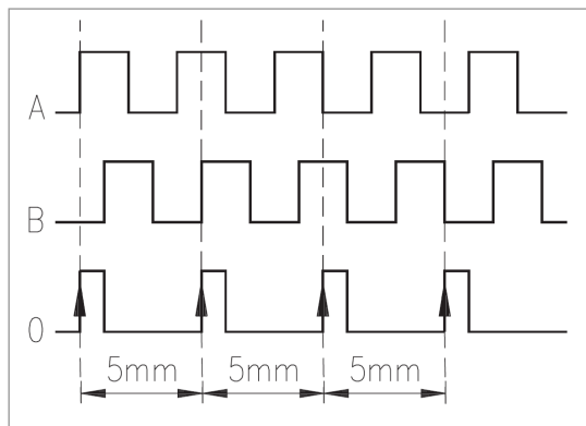
Abb. 3: Ausgangssignale A und B mit Referenzsignal (1 Inkrement)
