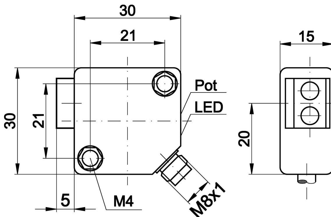
Massbild
