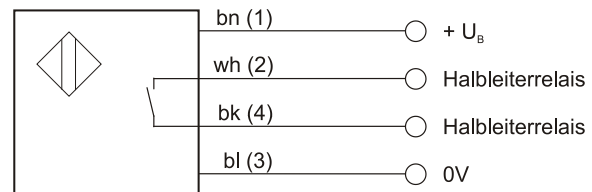
bn=braun, wh=weiß, bk=schwarz, bl=blau Klemmenbezeichnung der Kabeldose in Klammern
