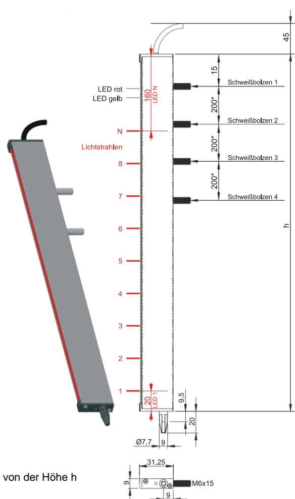
Bolzenbefestigung
