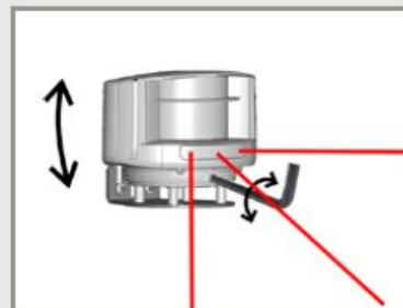
Falls notwendig, passen Sie den Neigungswinkel des Erfassungsfeldes mit einem Innensechskantschlüssel an.
