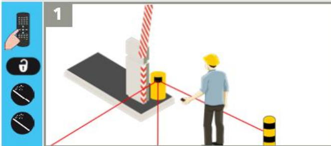
1 Die 3 sichtbaren Laserstrahlen mittels Fernbedienung aktivieren um den Sensor korrekt zu installieren.
