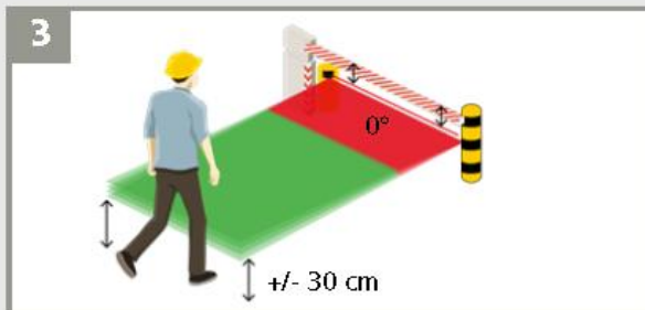
3 - Der 0° Strahl muss parallel zum Schrankenbaum ausgerichtet sein. - Der Anfang des Öffnungsfeldes sollte auf halber Beinöhe sein.
