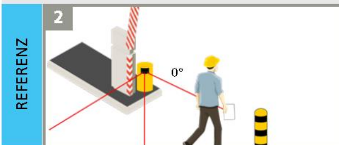
2 Mit Hilfe eines weißen Blatts können Sie die Position des 0° Laserstrahls prüfen. Der Referenzpunkt kann auf jedes Objekt angepasst werden, entweder am Ende des Schrankenbaums oder weiter weg. Die Oberfläche muss ca. 10 cm groß und fest verankert sein. Den reflektierenden Aufkleber benutzen, falls der Abstand zwischen Referenzpunkt und Sensor größer als 5 m ist.
