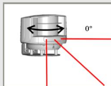
Falls notwendig, den Sensor leicht um seine Achse drehen, um den 0° Laserstrahl auf den Referenzpunkt anzupassen.
