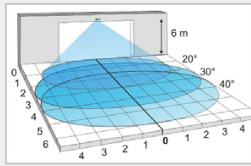
Montagehöhe: 6 m Boost-Funktion: ON Werkseinstellungen
