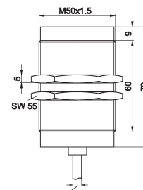
Silikonkabel Ø 5mm Teflonkabel Ø 3mm
