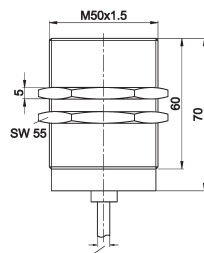
Silikonkabel Ø 5mm Teflonkabel Ø 3mm
