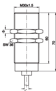
Silikonkabel Ø 5mm Teflonkabel Ø 3mm
