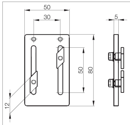
Maßskizze 2 (Montage in Profilen mit Nutenstein 12)
