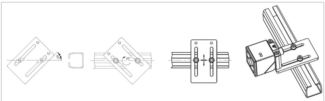
Montageanleitung (Beispiel)
