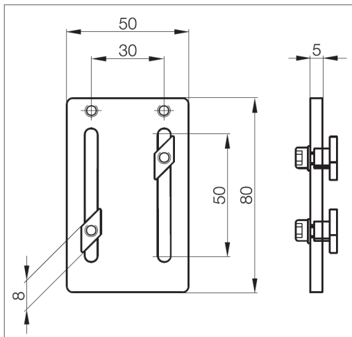
Maßskizze 1 (Montage in Profilen mit Nutenstein 8)
