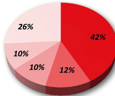
Einsparpotenziale bei der Druckluftherzeugung: 42%: Identifizierung und Beseitigung von Leckagen 12%: Auslegung des Pneumatiksystems einschließlich eines Mehrdruck-Leitungsnetzes 10%: Wärmerückgewinnung. 10%: Kompressoren mit variabler Motordrehzahl 26%: sonstige Maßnahmen
