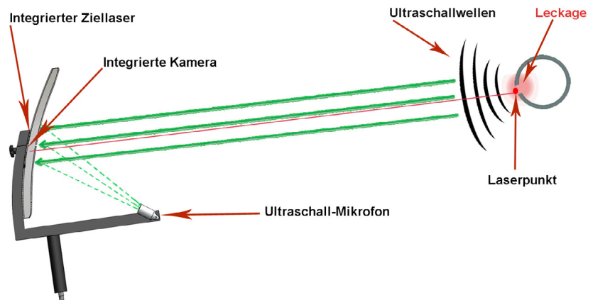
Funktionsweise des Parabolspiegels.
