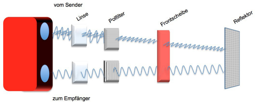
Funktion eines Polfilters. Der Filter der Sendeoptik ist nur für eine bestimmte Schwingungsachse des Lichts durchlässig. Ebenso verhält es sich mit dem empfängerseitigen Filter.
