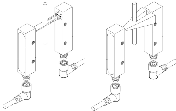
Links eine Laser-Lichtschanke, rechts eine konventionelle Lichtschanke.
