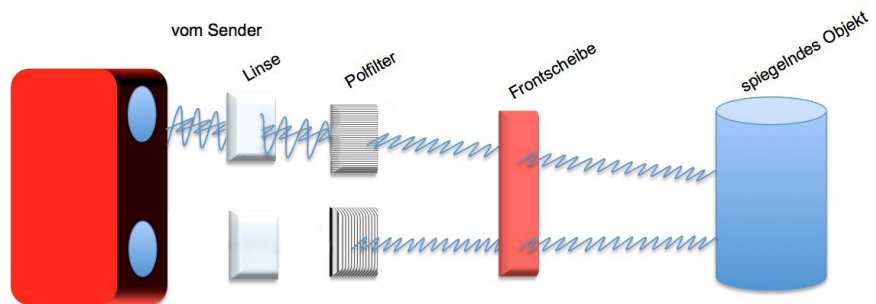
Das vom Objekt reflektierte Licht kann den Polfilter nicht passieren, so dass das Objekt sicher erkannt wird.
