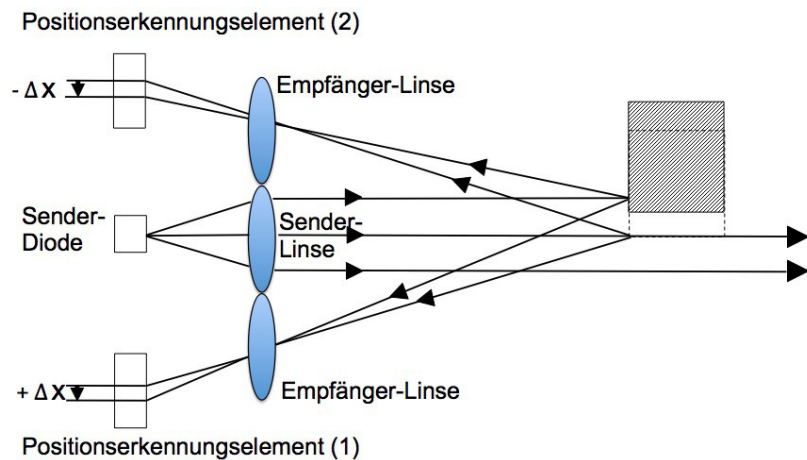
Funktionsweise der Hintergrundaussblendung nach dem Dreistrahlprinzip.
